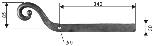
掛けガネ 439.04.000
