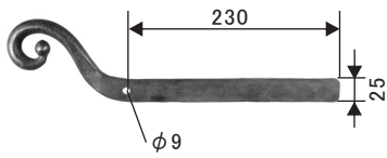
掛けガネ 438.04.000
