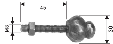
396.03.000
