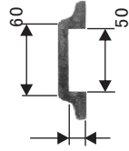
ストッパー 436.04.000
