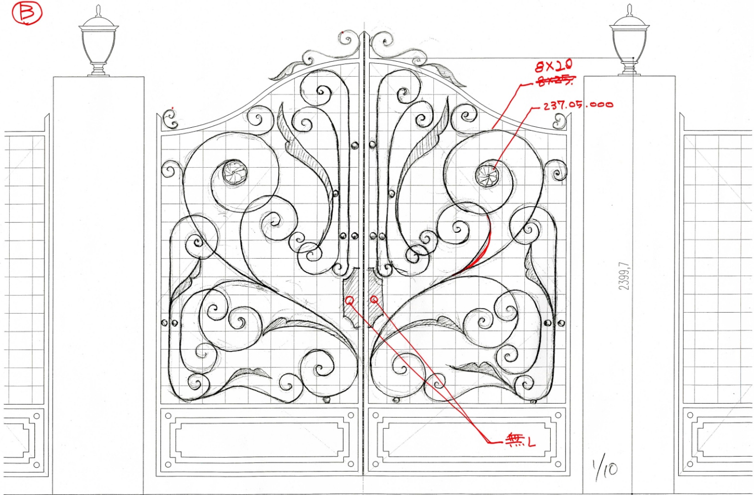
正面門扉
