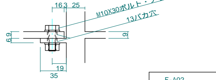
ジョイント詳細 1:3
