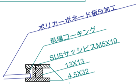
屋根板止め棧詳細 1:3
