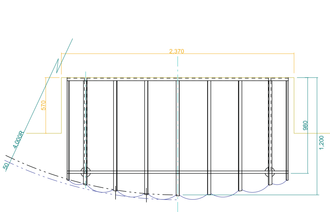
屋根板止め棧詳細 1:3
