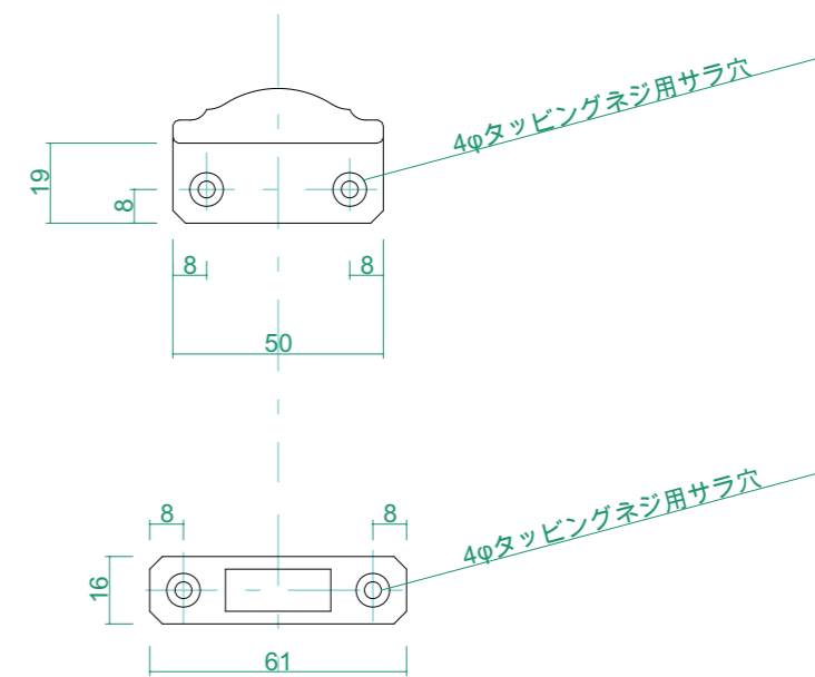
壁付BPL詳細 1:2
