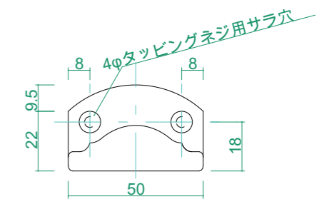
壁付BPL詳細 1:2
