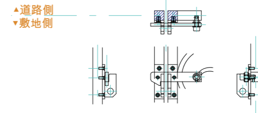
掛金詳細 1:10
