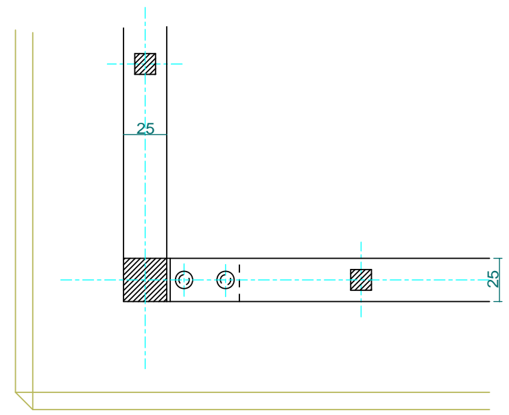
ボトムレールジョイント部詳細
