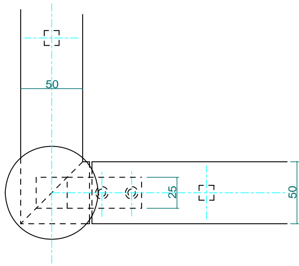
ハンドレールジョイント部詳細
