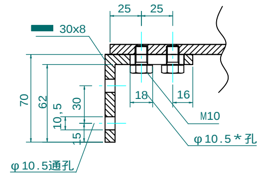
上部取付金具詳細 1:3
