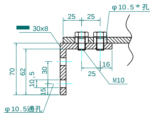
下部取付金具詳細 1:3
